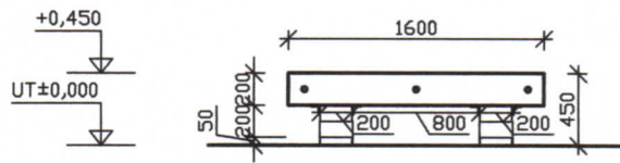
REZ - POZDĹŽNY:
